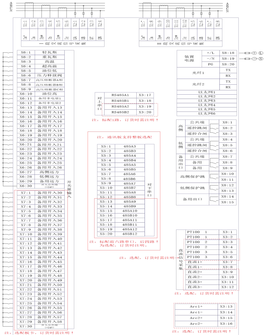
箱变智能测控装置接线图
