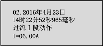
图 5.4-6 事故记录画面图
